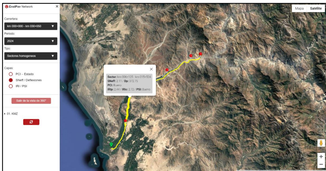
Figura 37 - Sectores Homogeneos de Sneft/Deflexiones en georreferencia
