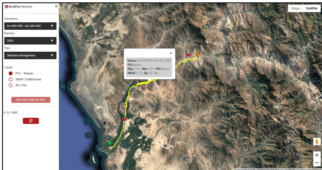
Figura 36 - Sectores Homogeneos de PCI – Estado en georreferencia
